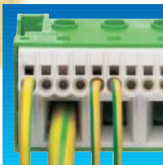
Le bornier de terre peut recevoir des conducteurs jusqu'à 25 mm 2
